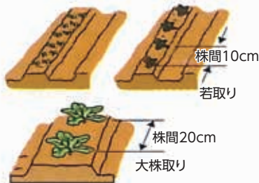
図4 追肥
