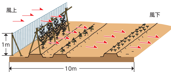
図2 防風ネットの設置
